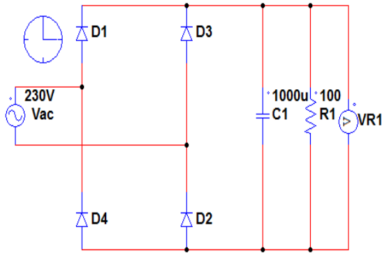
Fig: 2(a) AC-DC Rectifier
