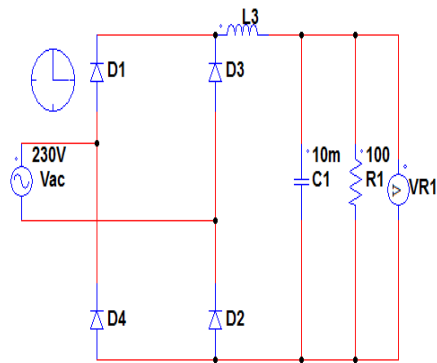
Fig: 3(a) AC-DC Filter Ckt.
